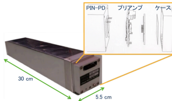
図 2.1: Belle II 実験電磁カロリメーターに使用されている CsI(Tl) カウンター。アルミ製のケース中に PIN-PD とプリアンプを収める
