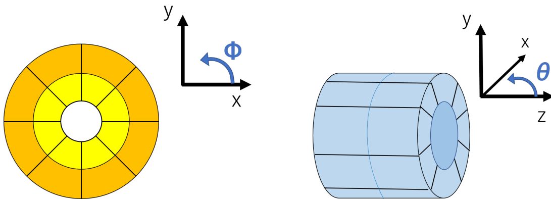
図 2.2: PIN-PD 電流値モニターの前方エンドキャップ 図 2.3: PIN-PD 電流値モニターのパレルを分割した図。
