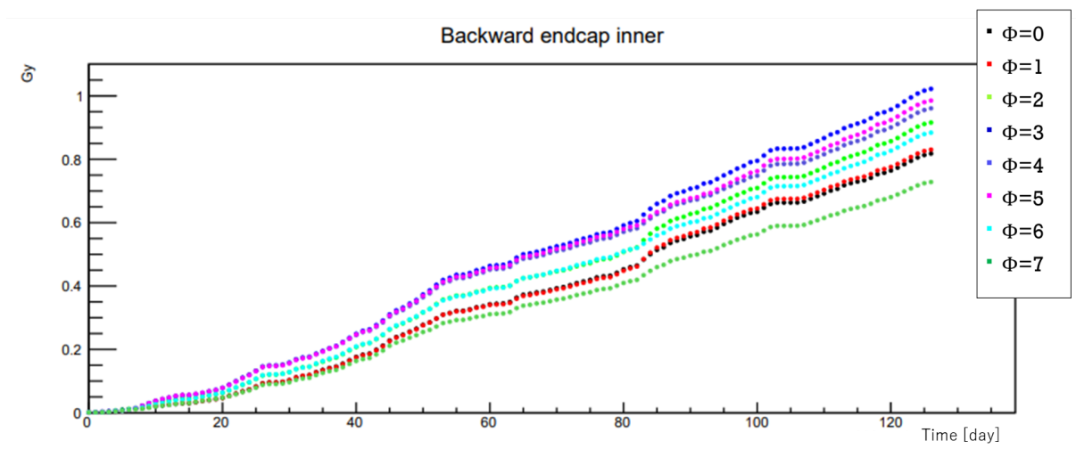
図 3.10: 後方エンドキャップ内側における放射線被ばく積算値
