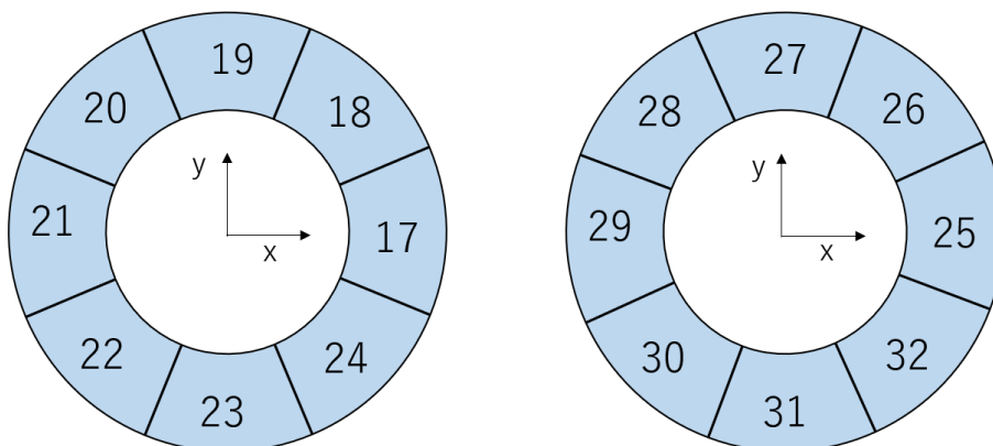
図 2.5: バレル前方 (左) と、後方 (右) におけるセグメントの位置とチャンネル番号
