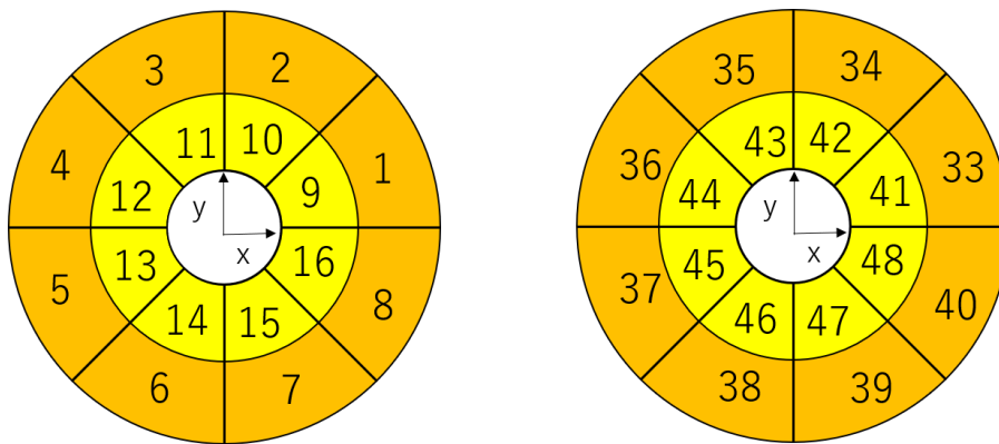
図 2.4: 前方エンドキャップ (左)、後方エンドキャップ (右) におけるセグメントの位置とチャンネル番号
