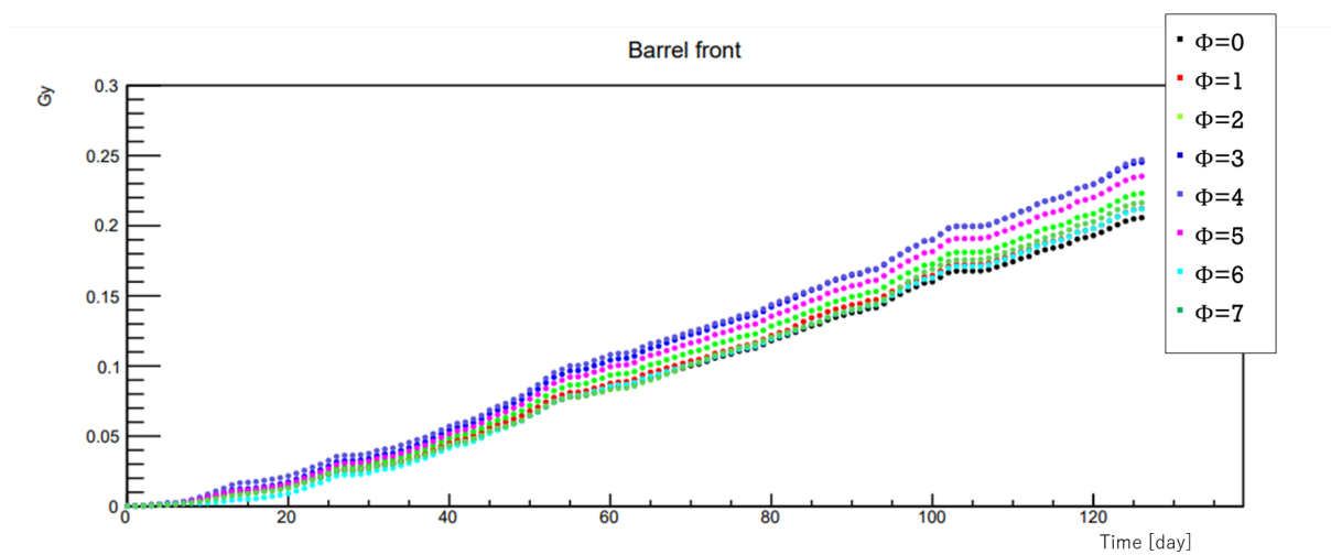
図 3.7: バレル前方における放射線被ばく積算値
